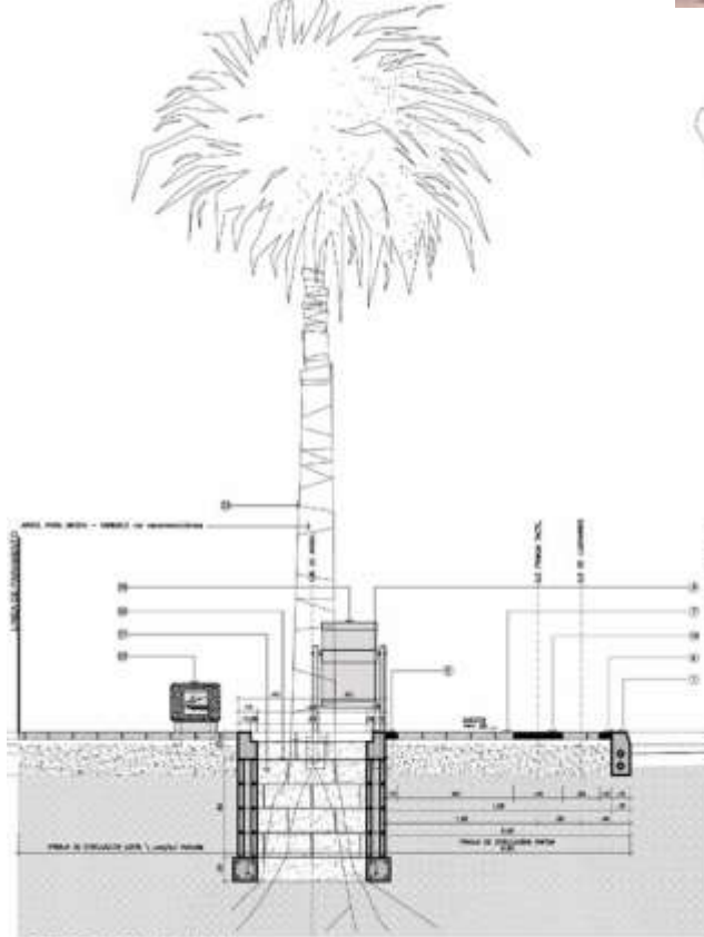
SECCION N-N DETALLE TÍPICO ÁRBOL EN TERRAZA A NIVEL TRAMO 1
