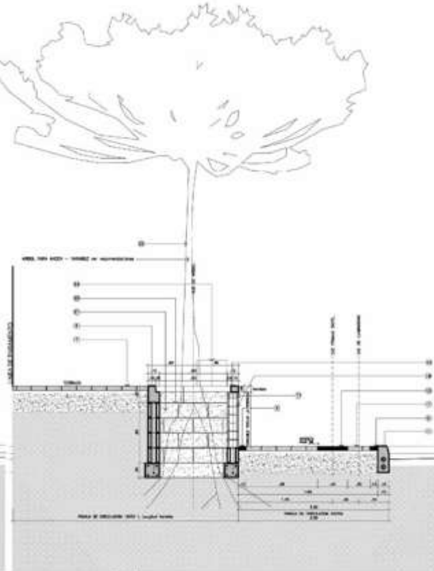
SECCION Ñ-Ñ DETALLE TÍPICO ÁRBOL EN TERRAZA ELEVADA TRAMO 1
